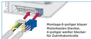
Abbildung 3.6.2-4: Montage blueMatic EV4/EAV4+ mit " Fingerscanner IDENCOM Biokey INSIDE, Mini X " (flügelseitig)
